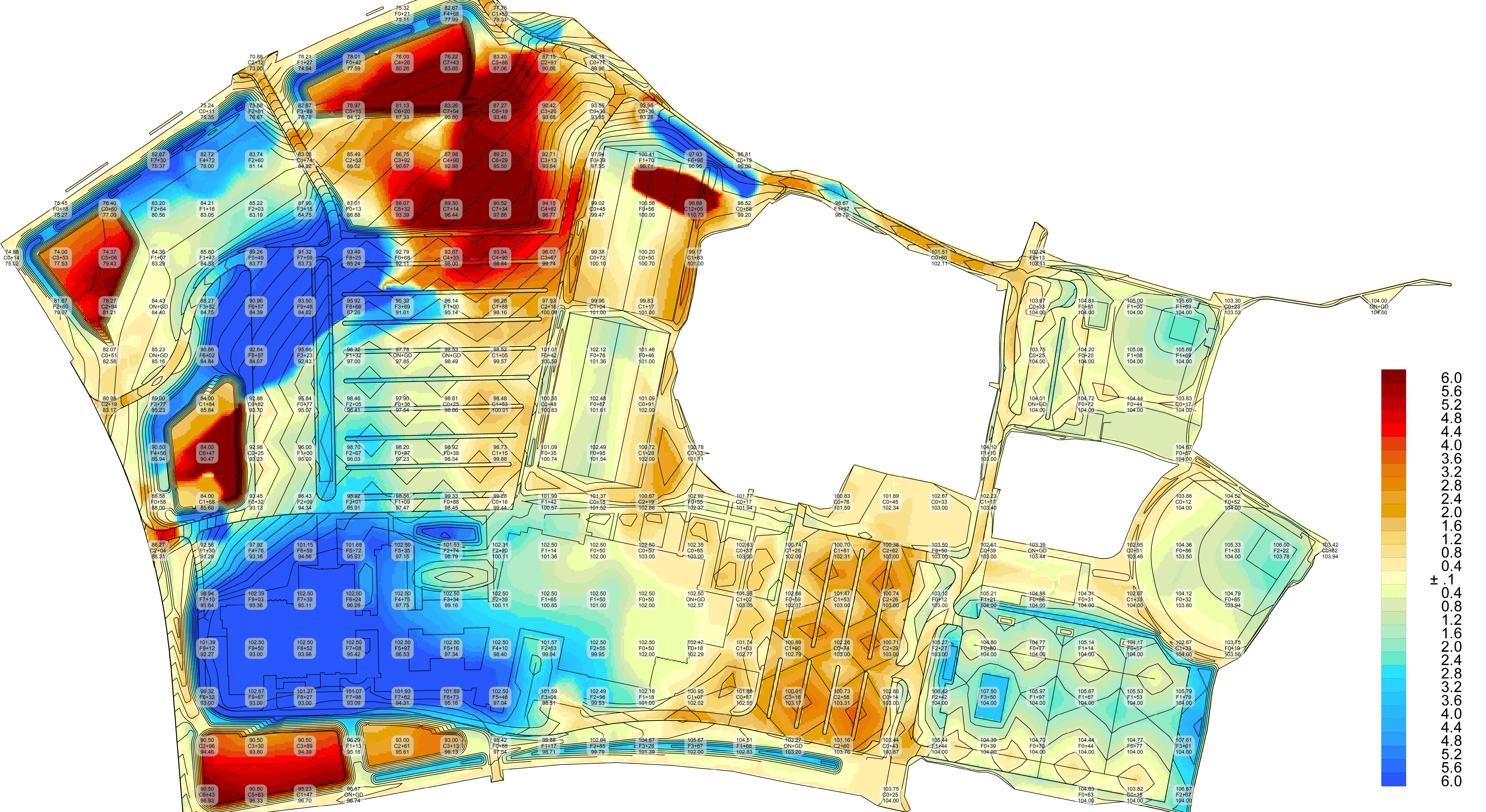
CUT FILL MAP
